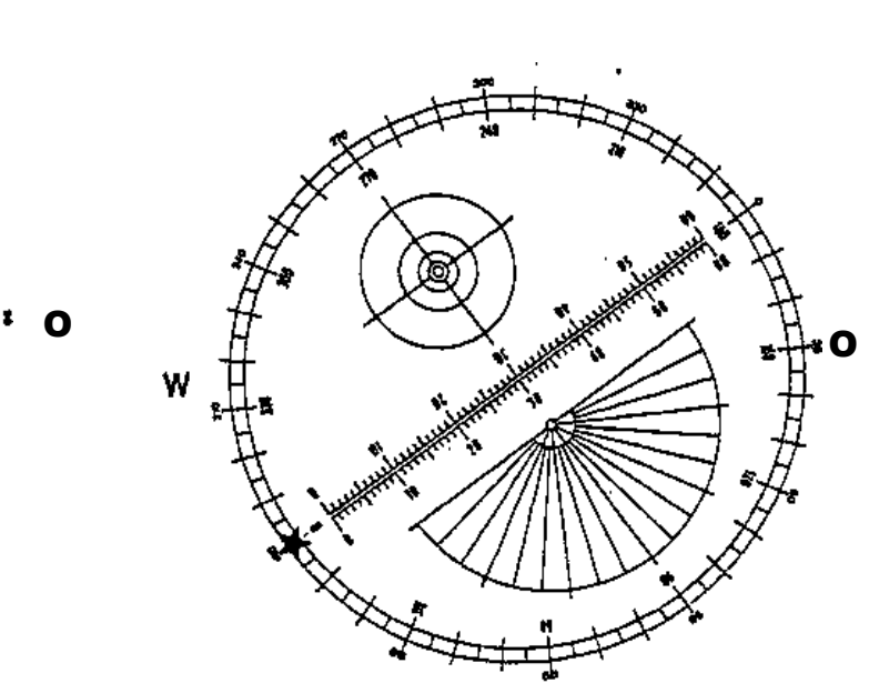
mit Zenitprisma
